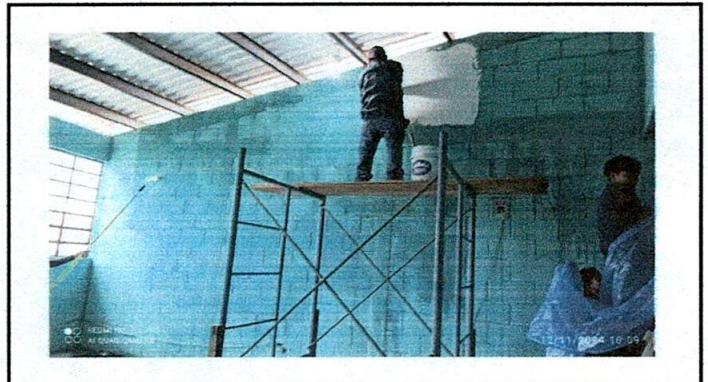
FOTO 10: REPELLO DE MUROS Y PAREDES
